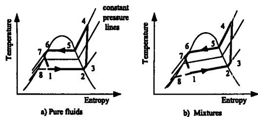
Fig. 4 : Vapour compression cycle on T-s plane
